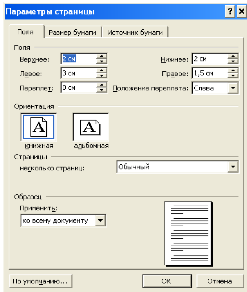
Рис. 4.1. Параметры страницы
