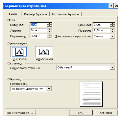
Рис. 5.1. Параметры страницы
