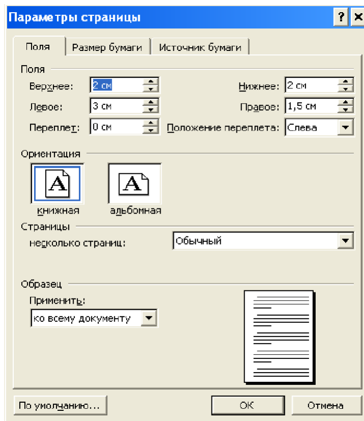
Рис. 4.1. Параметры страницы
