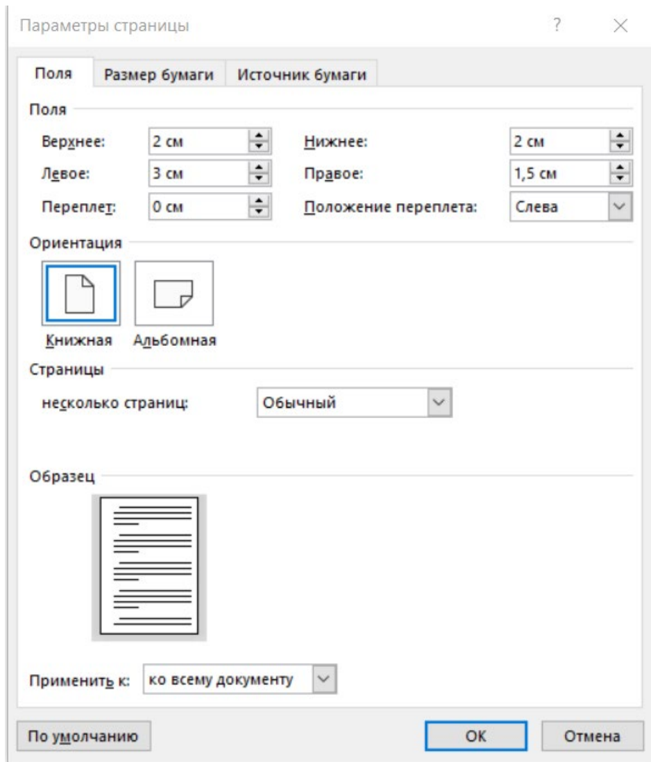
Рис. 5.1. Параметры страницы
