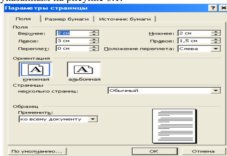
Рис. 6.1. Параметры страницы
