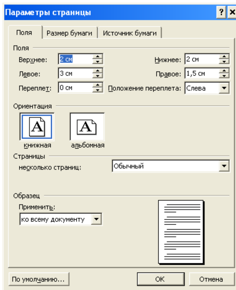
Рис. 5.1. Параметры страницы
