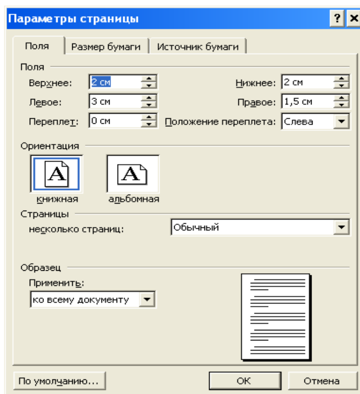
Рис. 7.1. Параметры страницы
