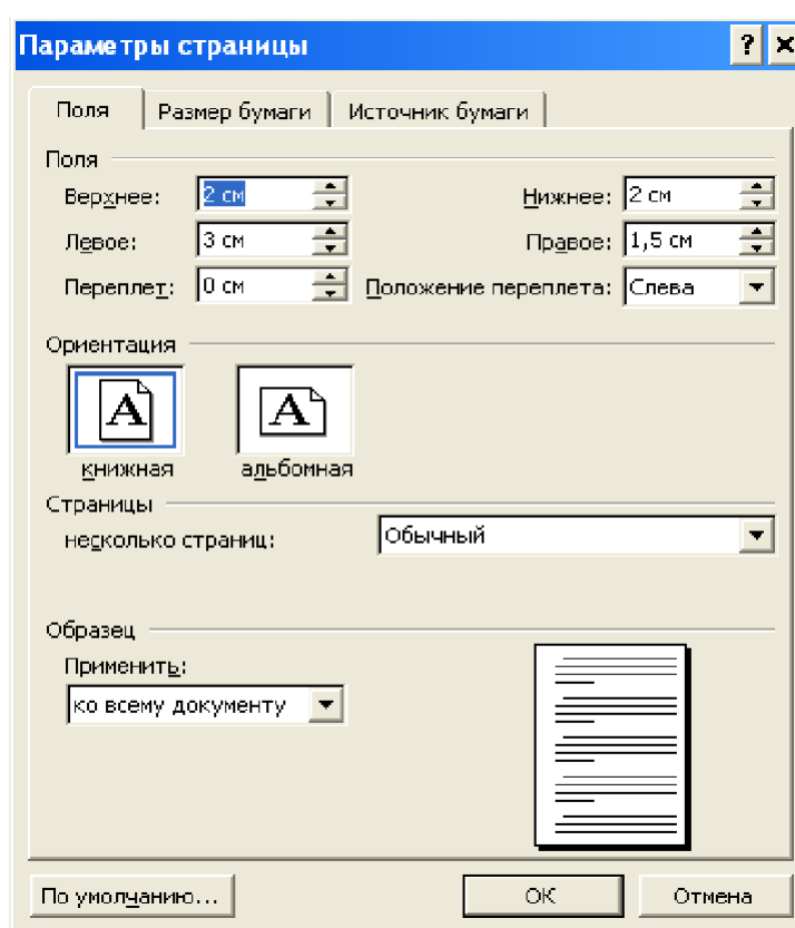
Рис. 4.1. Параметры страницы
