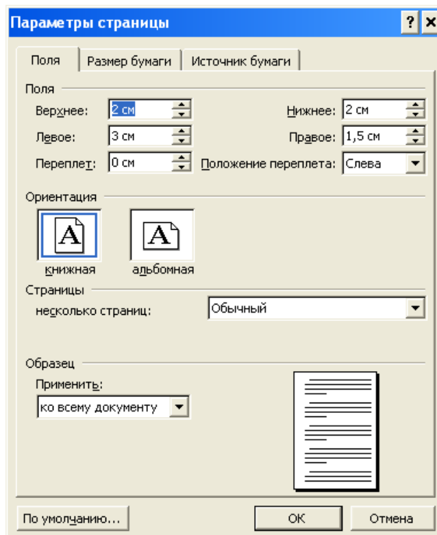
Рис. 5.1. Параметры страницы
