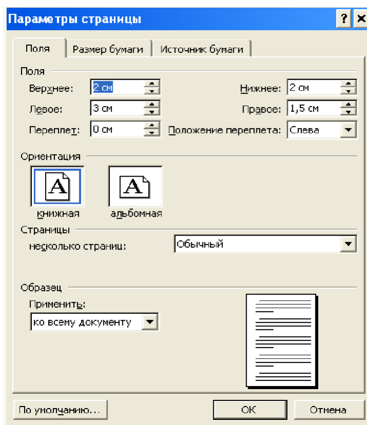
Рис. 6.1. Параметры страницы
