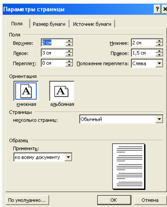
Рис. 5.1. Параметры страницы
