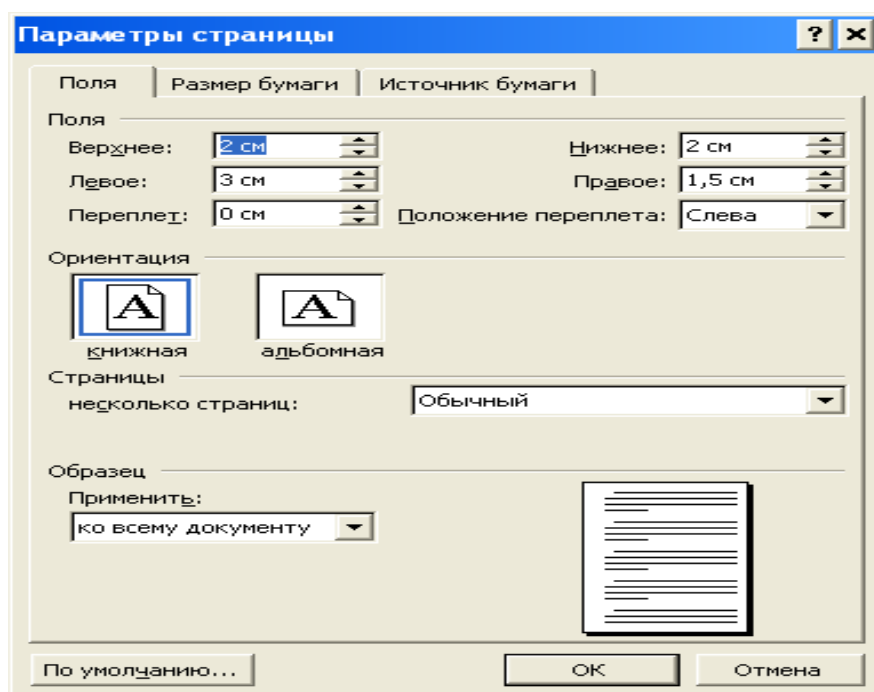
Рис. 3.1. Параметры страницы
