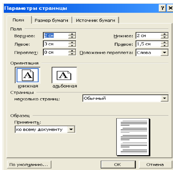
Рис. 6.1. Параметры страницы
